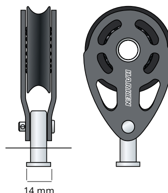
KUN 57 + 75 mm MASTEFODSBLOK
