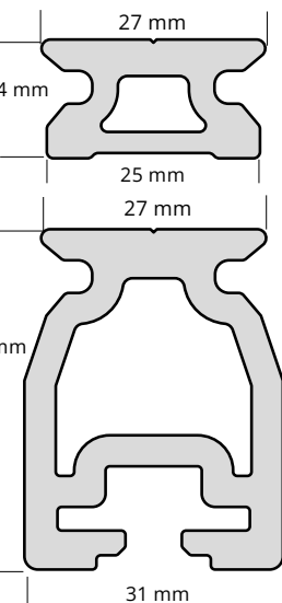
HK-T2721B-HL
