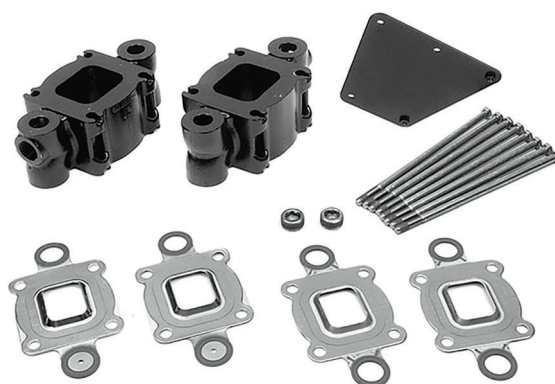
Risersæt til manifold 18-1842, 18-1843
