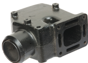
3" til manifold 18-1952-1, 18-1953-2, 18-1957-2
