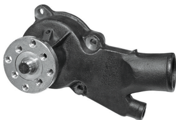
GM 4 &amp; 6 cyl. rækkemotor
