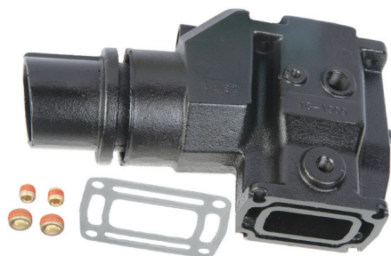
4" til manifold 18-1848, 18-1986-1
