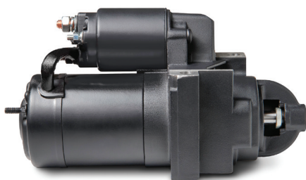
12V, 11 tænder, forskudte bolte GM 4.3L 1996- & 5.0 / 5.7L 1998- m. 14" svinghjul
